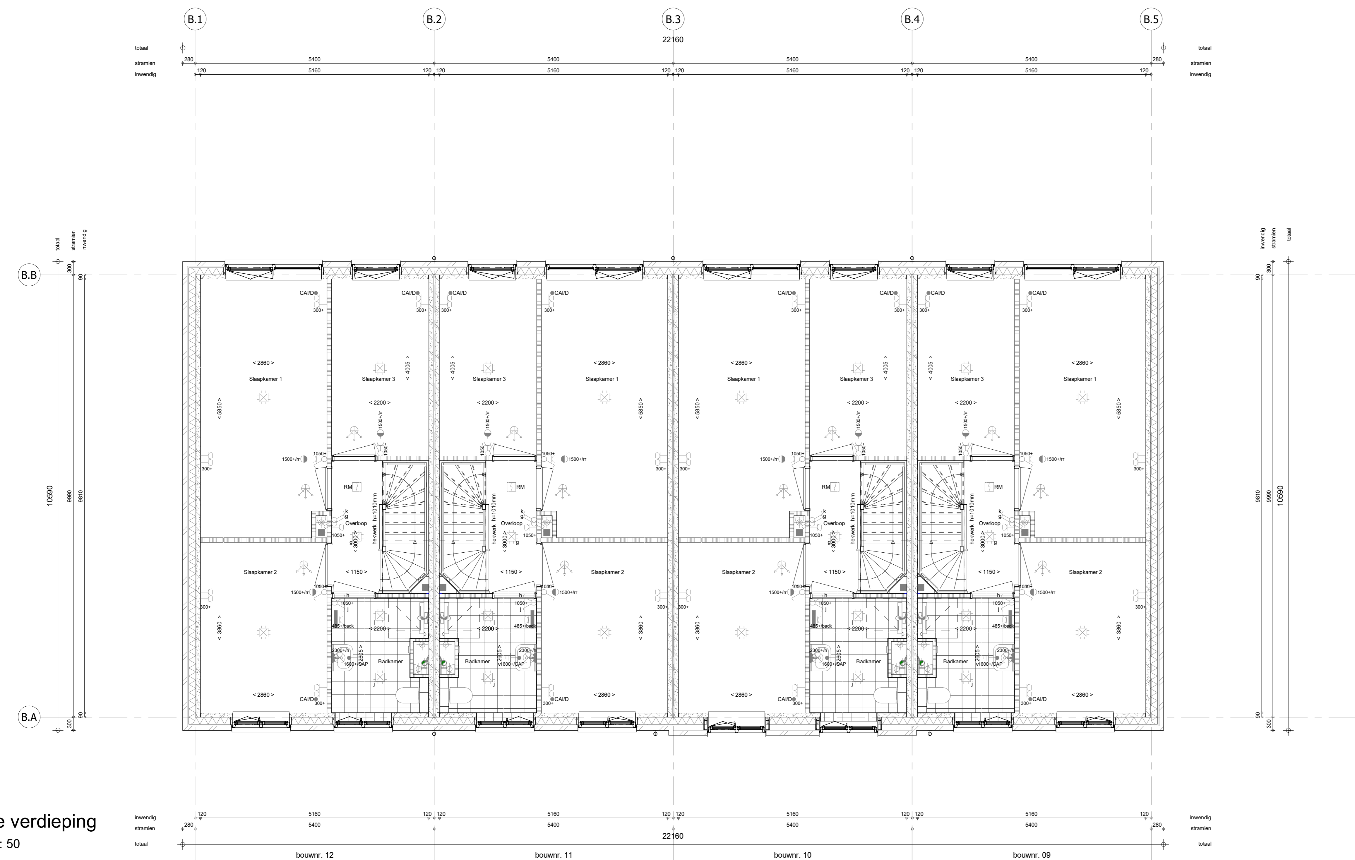
Begane grond 1 : 50
